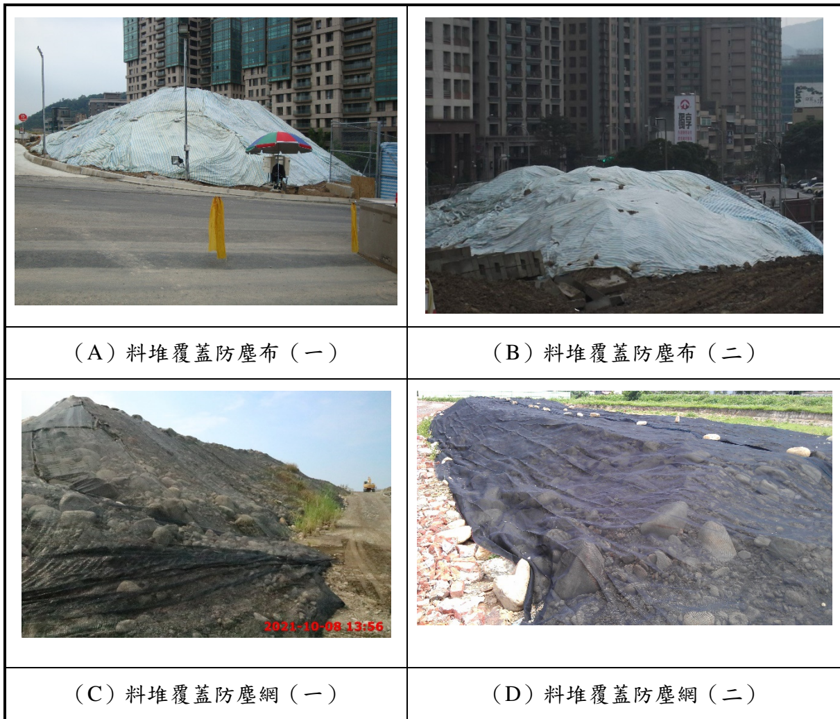
圖十一 營建工地堆置具粉塵逸散性之工程材料、砂石土方或廢棄物時，所應採行之防制設施內容及標準
