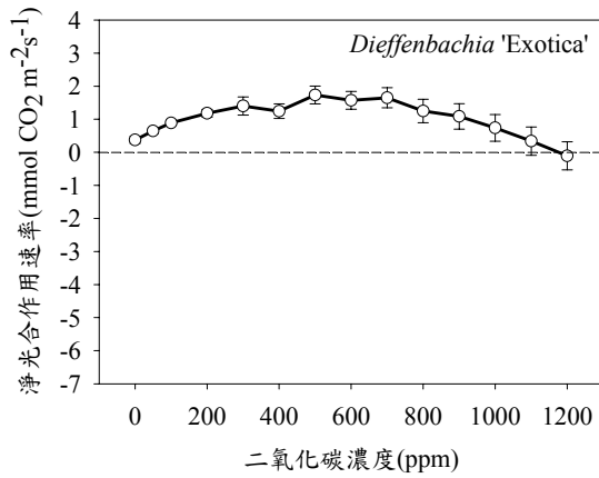
▲黛粉葉在室內二氧化碳濃度 0-1100 ppm 範圍內，有淨光合作用，可減少二氧化碳。
