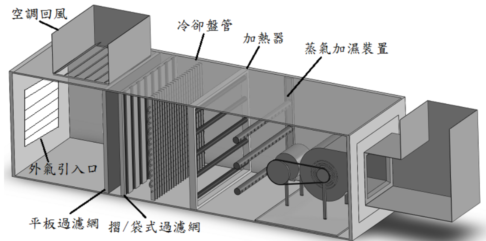
圖 6 外氣引入與空調箱混合型式示意圖
